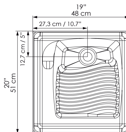
VISTA EN PLANTA / UPPER VIEW
