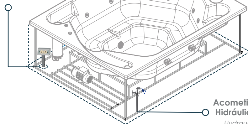
Acometidas Eléctricas Electric connections
