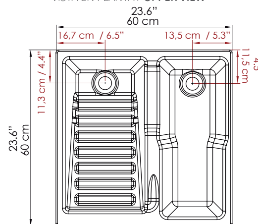
VISTA EN PLANTA / UPPER VIEW
