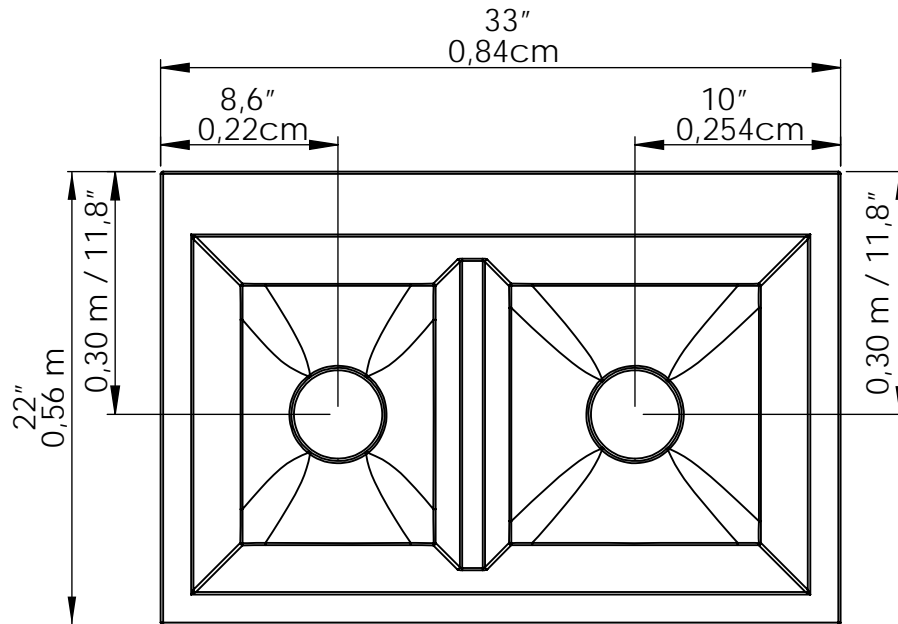
VISTA EN PLANTA / PLANT VIEW
