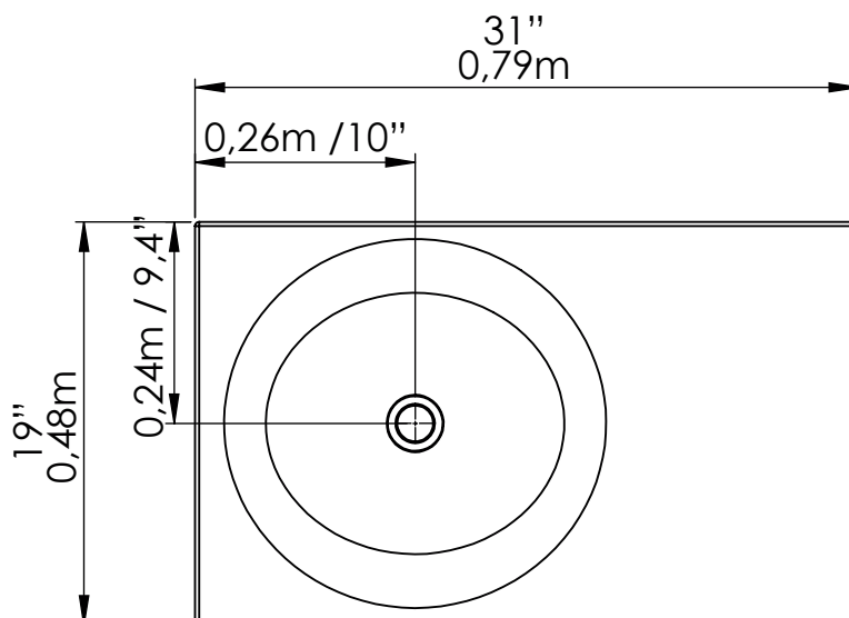
VISTA EN PLANTA / UPPER VIEW
