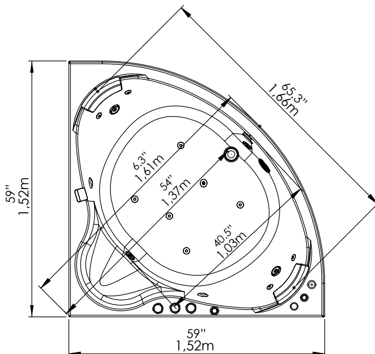
VISTA EN PLANTA / UPPER VIEW
