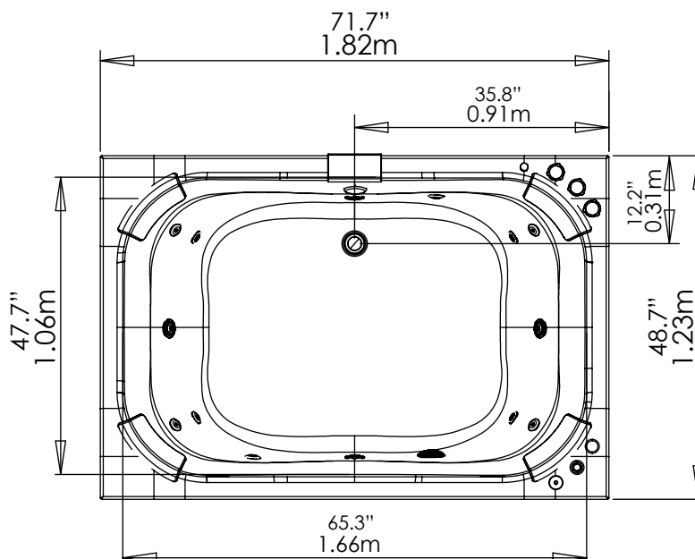
VISTA EN PLANTA / UPPER VIEW
