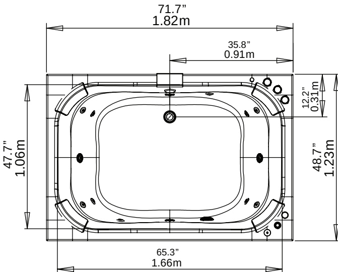
VISTA EN PLANTA / UPPER VIEW
