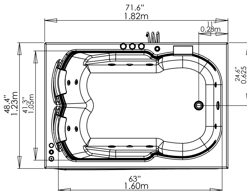
VISTA EN PLANTA / PLANT VIEW
