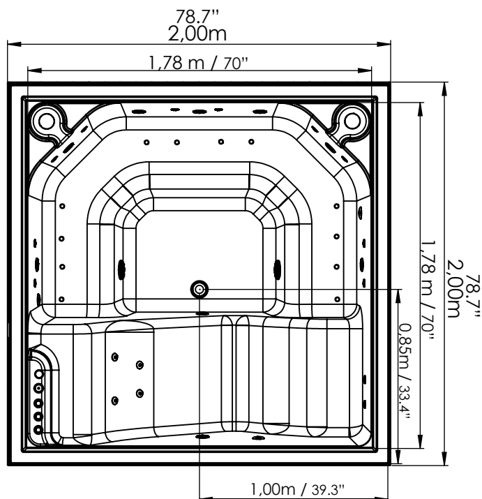
VISTA EN PLANTA / UPPER VIEW
