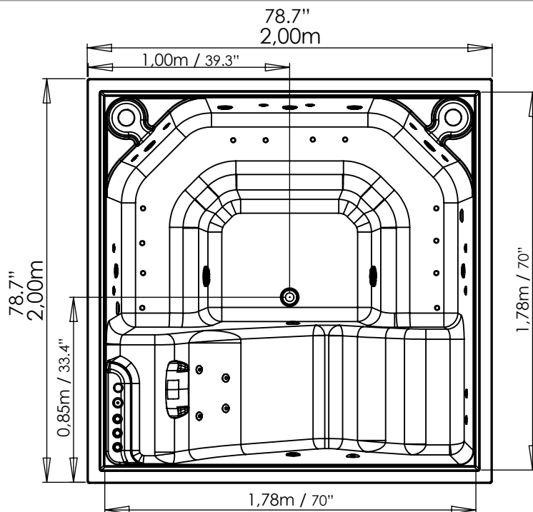
VISTA EN PLANTA / UPPER VIEW
