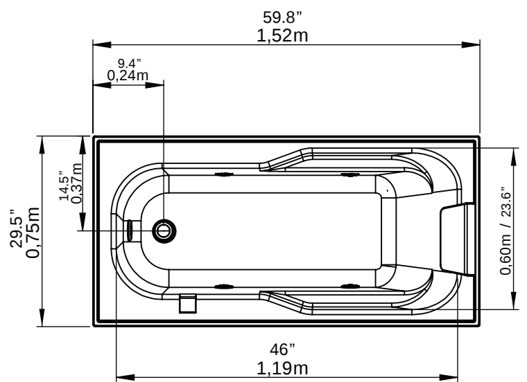
VISTA EN PLANTA / PLANT VIEW
