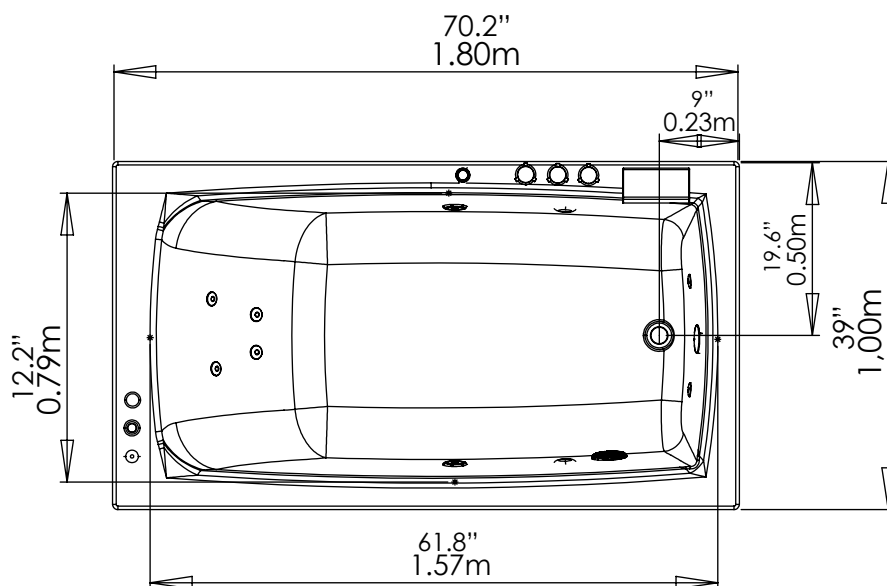
VISTA EN PLANTA / PLANT VIEW
