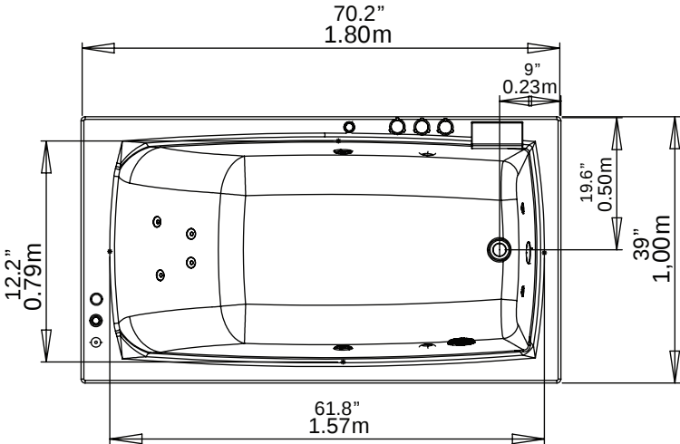
VISTA EN PLANTA / PLANT VIEW
