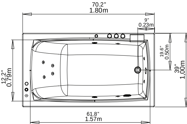
VISTA EN PLANTA / PLANT VIEW
