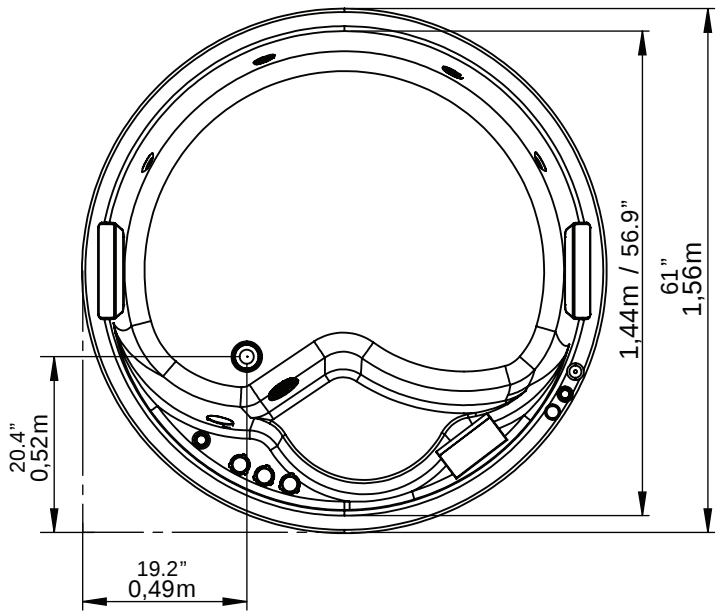
VISTA EN PLANTA / PLANT VIEW
