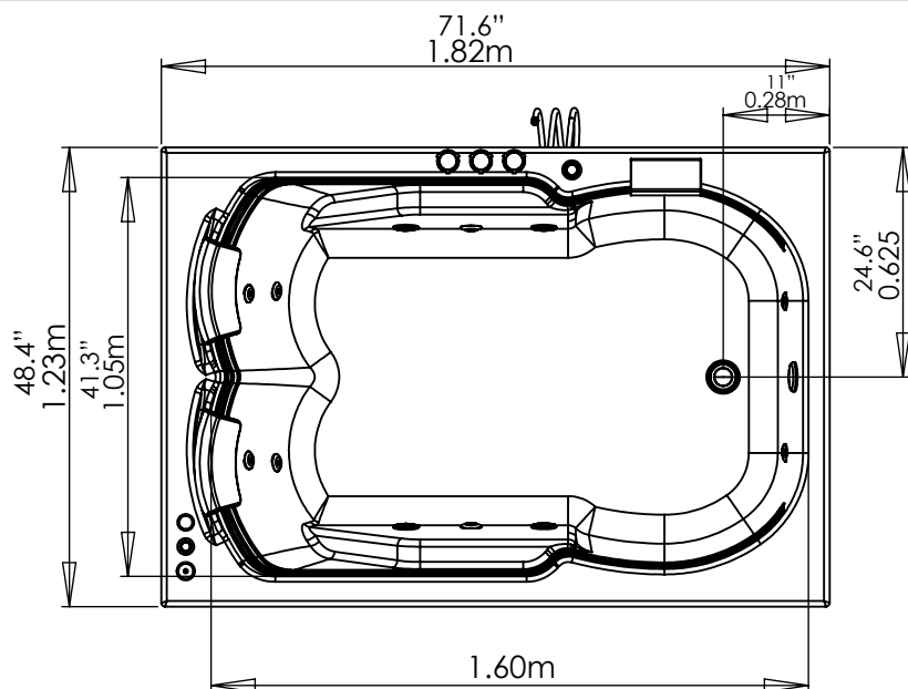
VISTA EN PLANTA / PLANT VIEW
