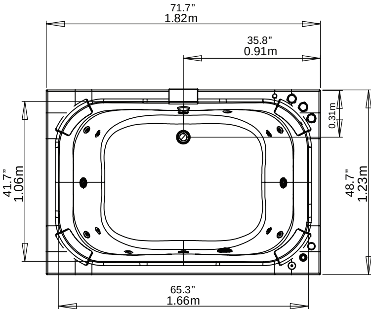
VISTA EN PLANTA / PLANT VIEW
