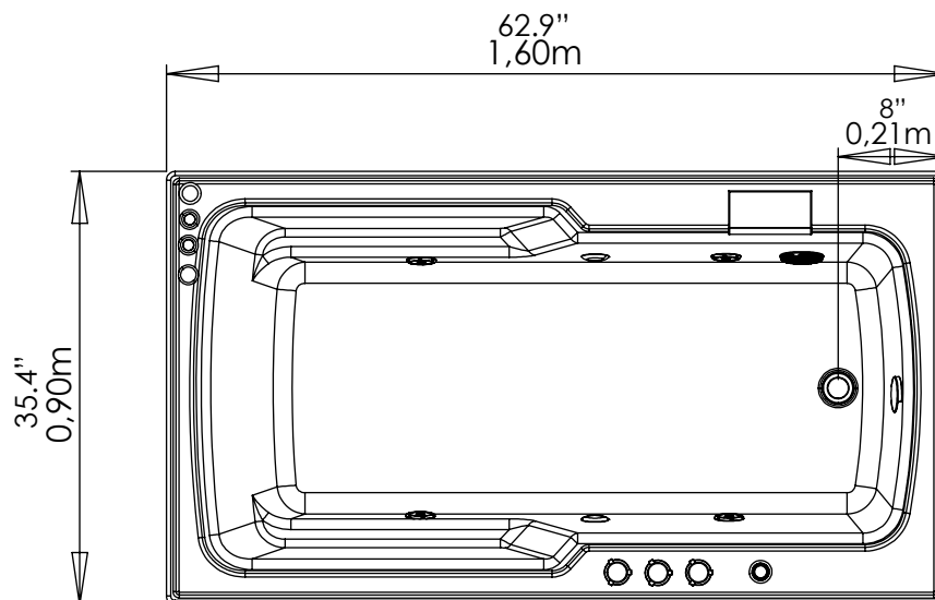
VISTA EN PLANTA / PLANT VIEW
