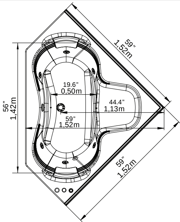
VISTA EN PLANTA / PLANT VIEW
