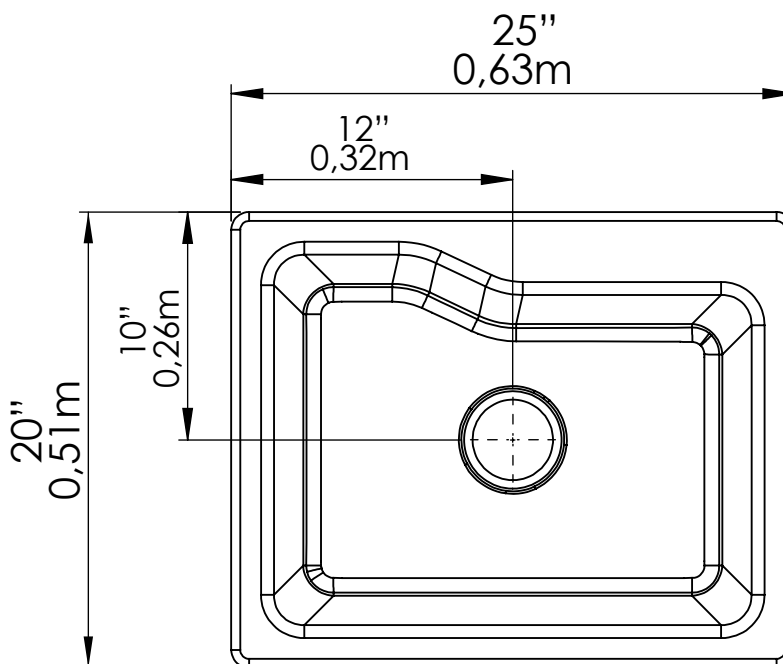
VISTA EN PLANTA / PLANT VIEW
